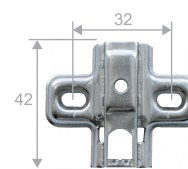
Base chapa H0 y H2
