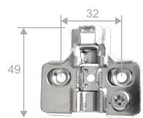
Base regulación excéntrica H0 y H2
