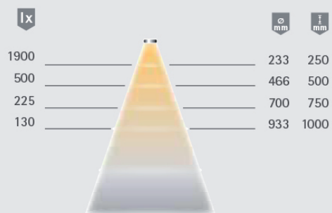
Diagrama de distribución luminosa 50°
