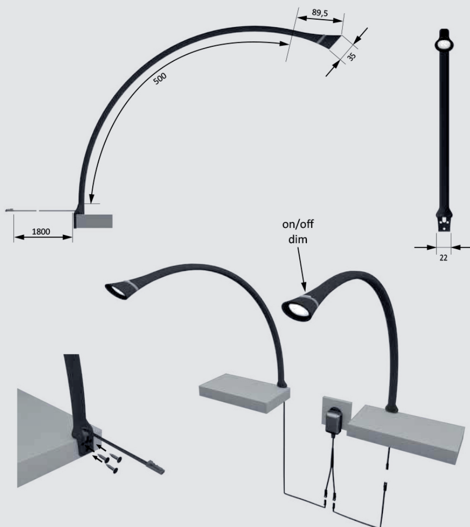
Esquema de montaje
