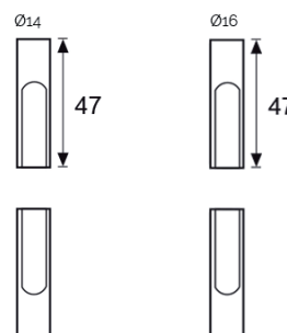
Plano de capuchones para pernio Anuba
