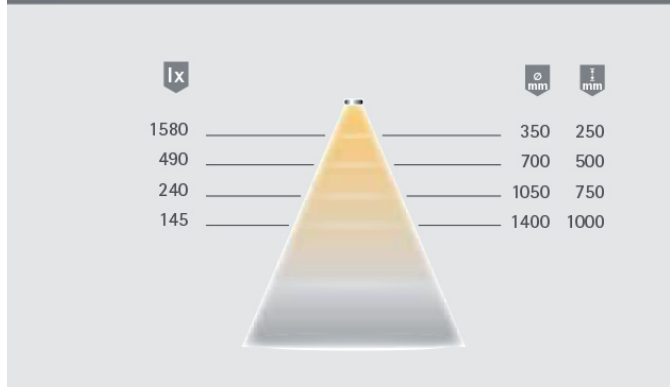
Diagrama de distribución luminosa 60°
